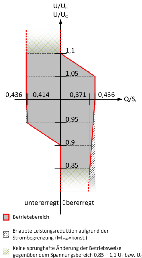
Abbildung 7-1: Blindleistungsbereich (Darstellung für die Niederspannung U/U_n bzw. für die Mittelspannung U/U_c bezogen auf einen Leistungsfaktor 0,9 bei Nennscheinleistung S_r mit Blindleistung Q=0,436 S_r )
