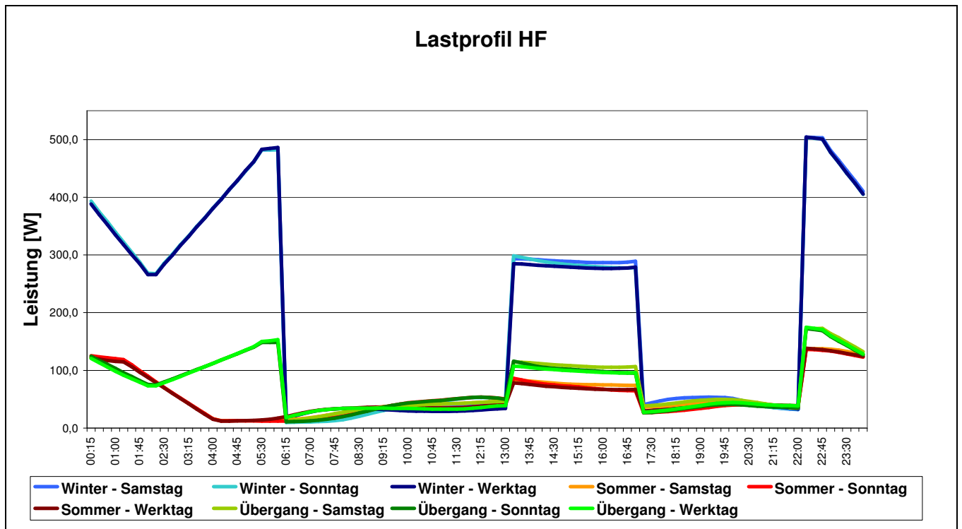
Abbildung 10: Lastprofil HF
