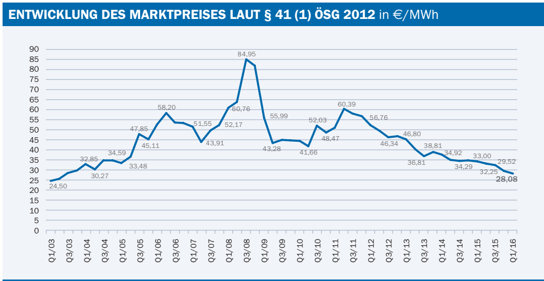
Abbildung 14 Entwicklung des Marktpreises laut § 41 (1) ÖSG 2012
