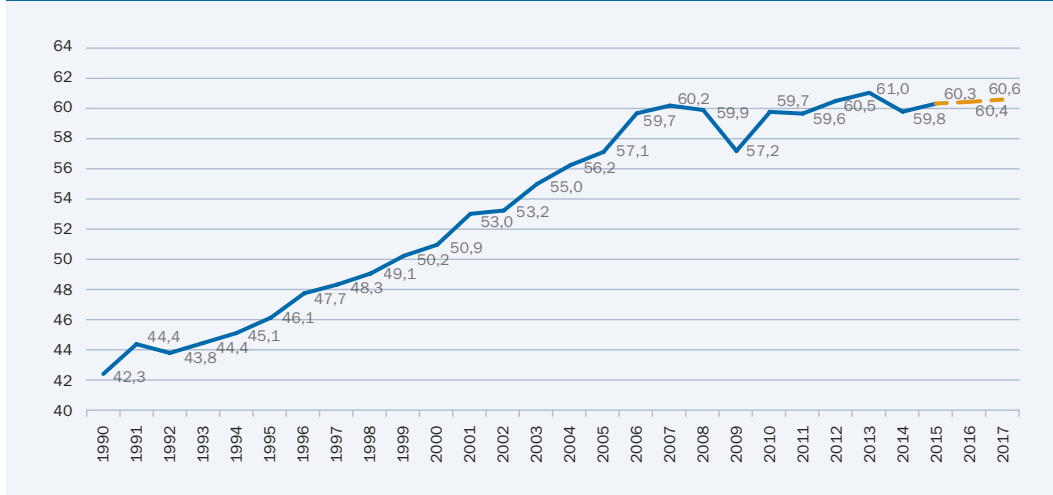
Abbildung 2 Stromverbrauch (energetischer Endverbrauch) von 1990 bis 2017 in TWh
