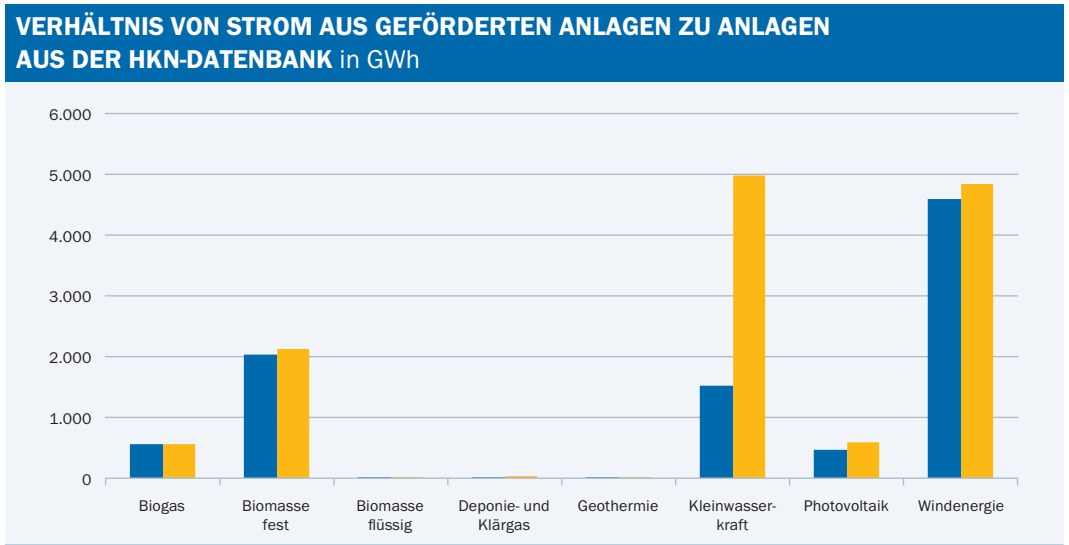
Abbildung 9 Verhältnis von Strom aus geförderten Anlagen zu Anlagen aus der HKN-Datenbank in GWh
