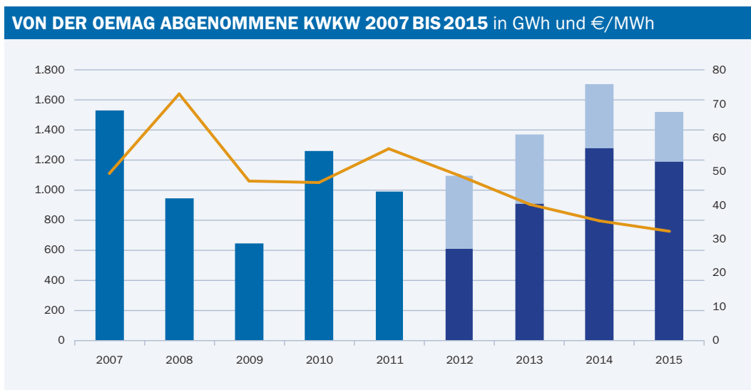
Abbildung 11 Von der OeMAG abgenommene KWKW 2007 bis 2015
