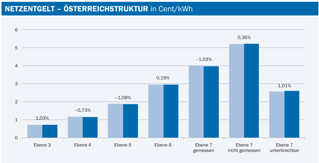
Abbildung 8 Netzentgeltentwicklung Österreichstruktur
