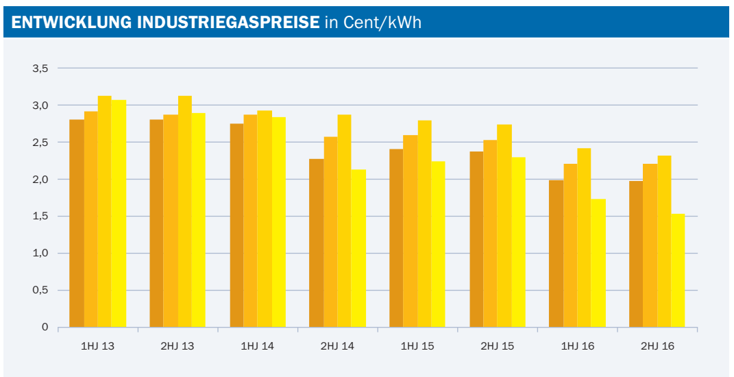
Abbildung 31 Entwicklung Industriegaspreise
