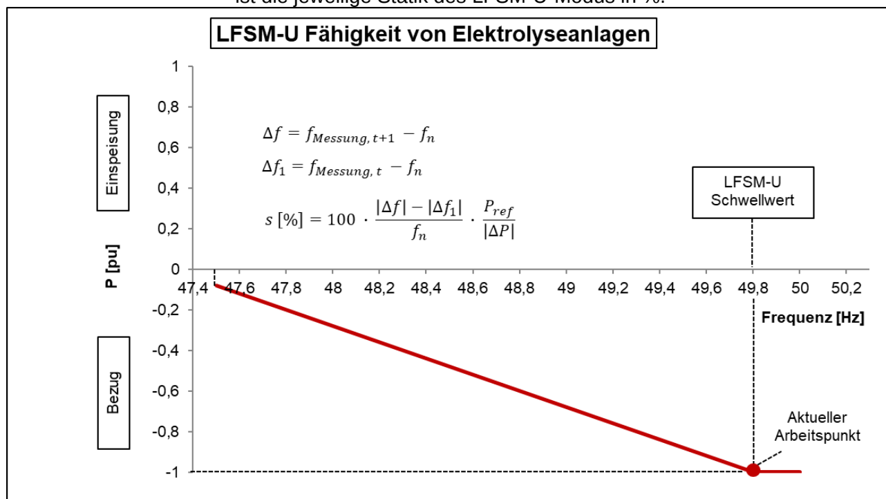
Abbildung 5: Fähigkeit von Elektrolyseanlagen zur frequenzabhängigen Anpassung der Wirkleistung im LFSM-U-Modus (Darstellung für P_{\text{ref}} = P_{\text{nom}} und s = 5 \% )
