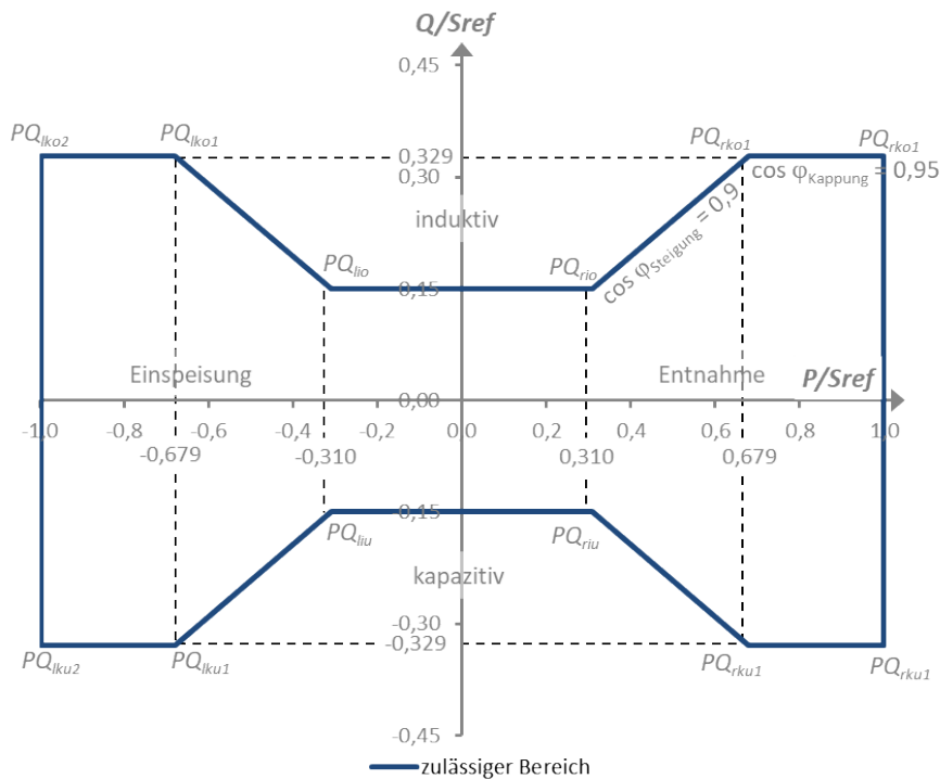
Abbildung 8: Zulässiger Blindleistungsbereich für Verteilernetze mit Verteilernetzanschluss ( Q ist die Blindleistung des Verteilernetzes in Mvar, P ist die Wirkleistung des Verteilernetzes in MW, S_{ref} ist die Referenzscheinleistung in Mvar und \cos \varphi ist der Verschiebungsfaktor.)
