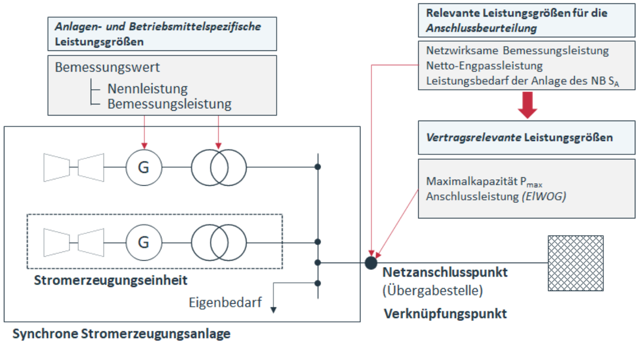
Abbildung 5: Schema Leistungsbegriffe synchrone Stromerzeugungsanlagen 1
