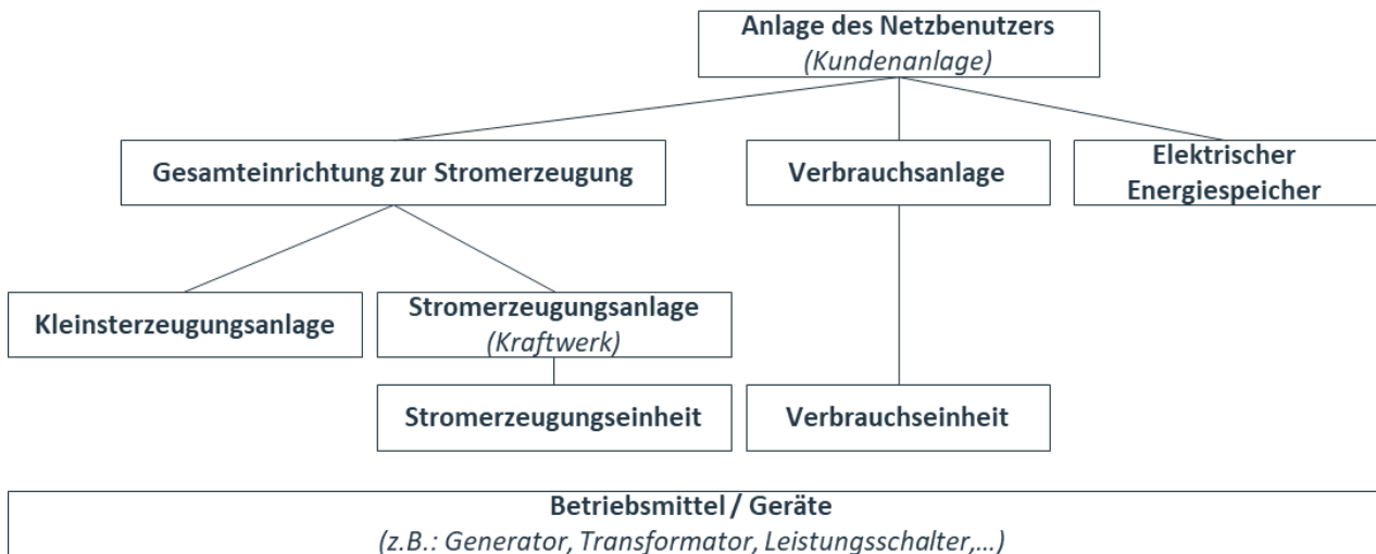
Abbildung 2: Schema Anlagenbegriffe Netzbewutzer
