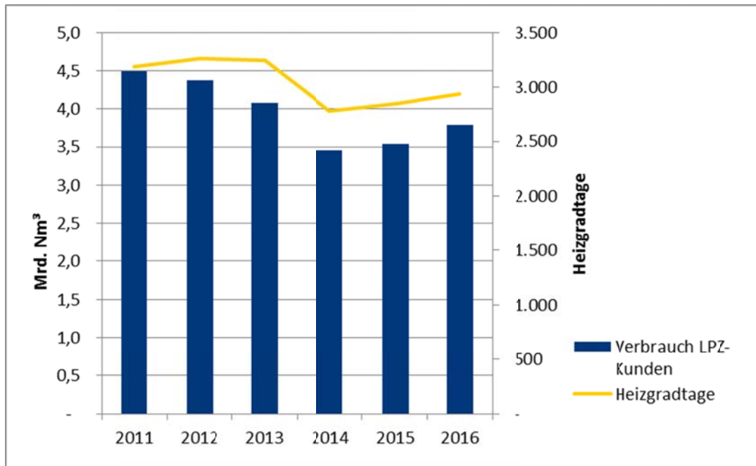
Diagramm 3: Verbrauch der LPZ Kunden von Oktober bis April und Heizgradtage absolut im Marktgebiet Ost in den Gasjahren 2011 bis 2016
