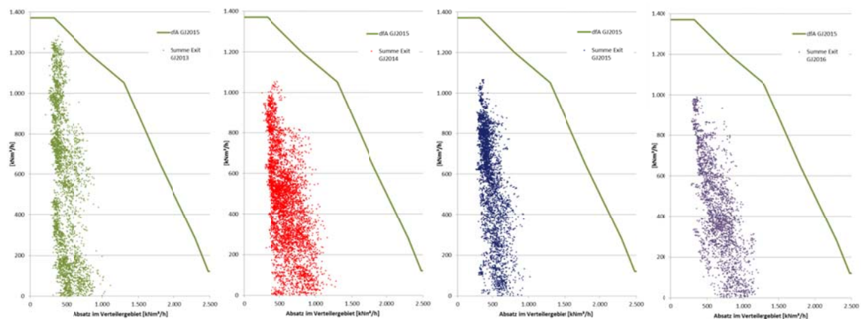
Diagramm 17: Vergleich der Exit Transporte aus dem Verteilergebiet in die Speicher (ohne Speicher Wien) in den Gasjahren 2013 bis 2016 (bis 1.6.2016)
