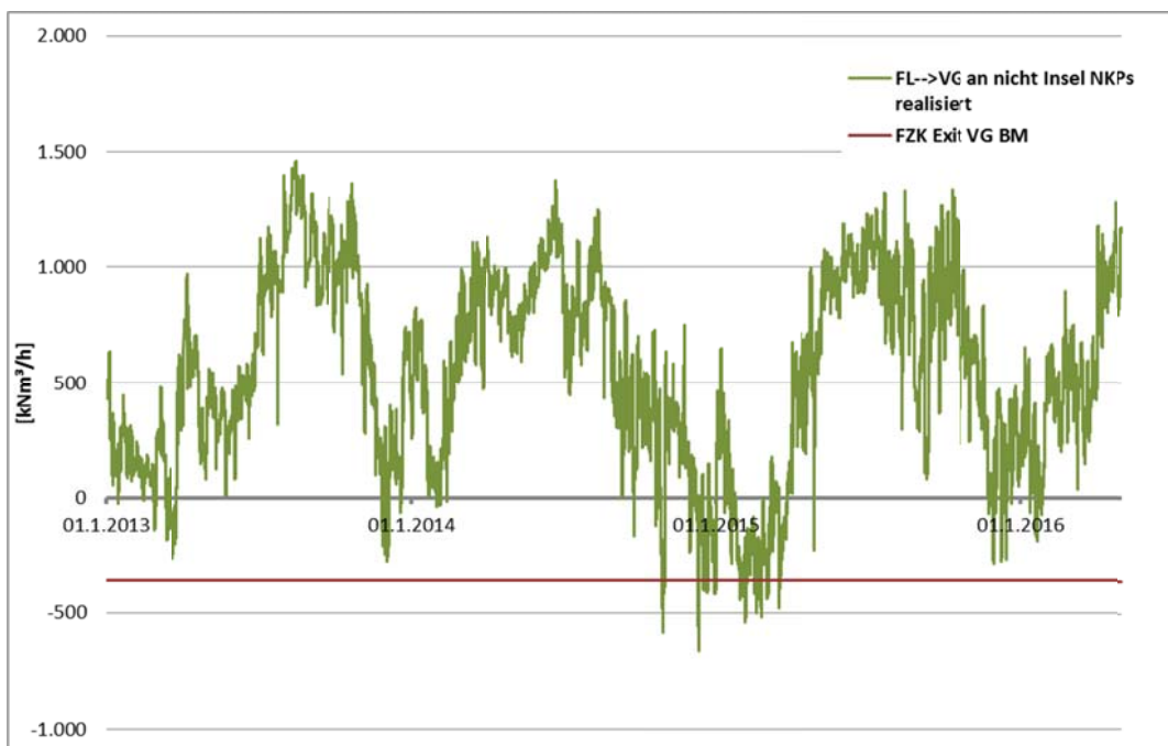
Diagramm 15: Transporte von der Fernleitungsebene in das Verteilerggebiet ohne TAG und WAG Insel Netzkoppelungspunkte und FZK Kapazität vom Verteilerggebiet in das Fernleitungsnetz
