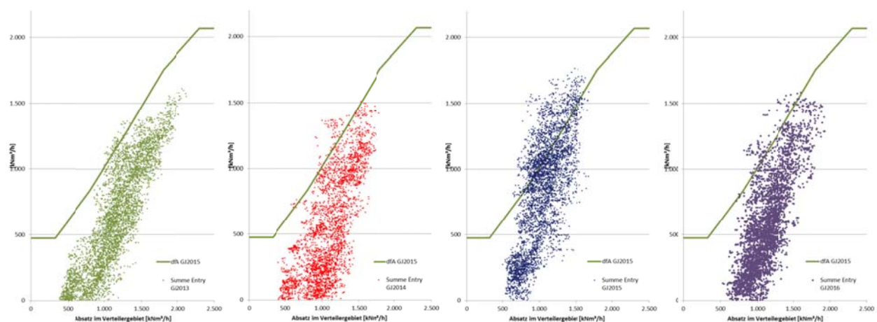
Diagramm 16: Vergleich der Entry Transporte aus den Speichern (ohne Speicher Wien) in das Verteilergebiet in den Gasjahren 2013 bis 2016 (bis 1.6.2016)
