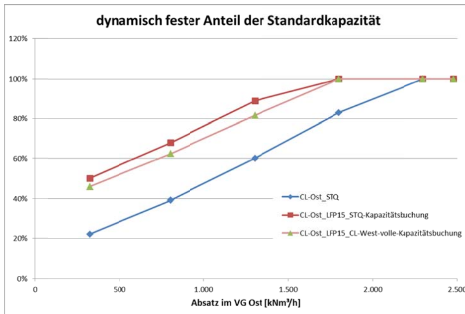
Diagramm 19: Dynamisch fester Anteil der Standardkapazität für den hydraulischen Cluster Ost im Status Quo und bei Umsetzung der genehmigten Projekte
