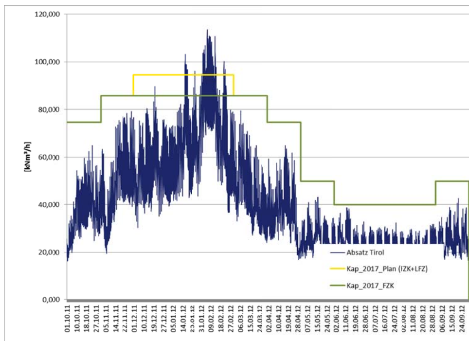
Diagramm 13: Absatz- und Kapazitätseingangsdaten für die Modellrechnung für das Marktgebiet Tirol
