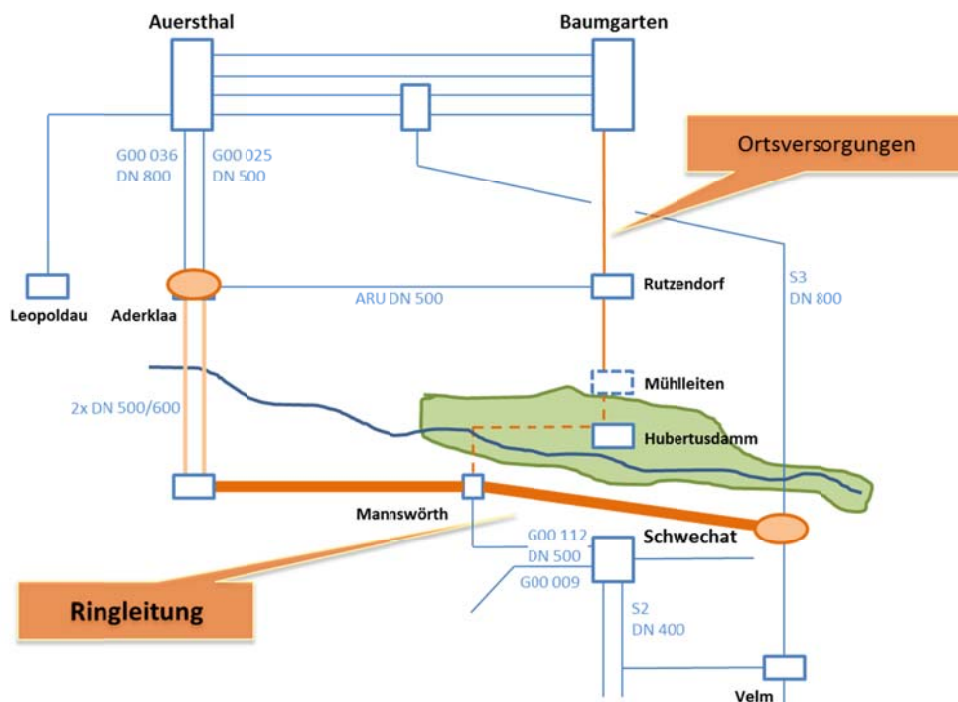
Abbildung 7: Projektidee Ringleitung
