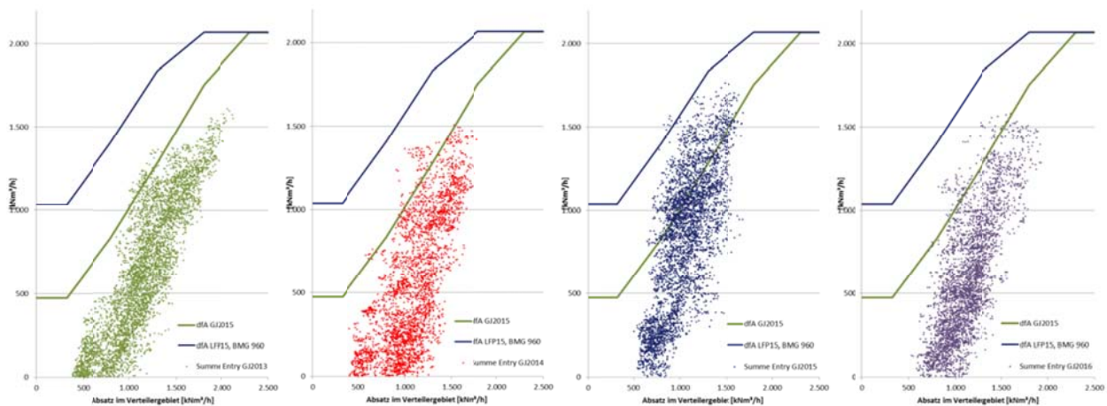
Diagramm 20: Vergleich der Entry Transporte aus den Speichern (ohne Speicher Wien) in das Verteilergesamt in den Gasjahren 2013 bis 2016 (bis 1.6.2016) und der dynamisch feste Anteil der Standardkapazität im STQ und nach Umsetzung der genehmigten Projekte bei derzeitiger Kapazitätsbuchung (1.6.2016)
