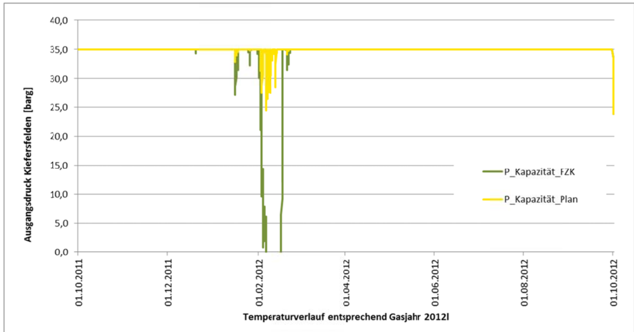
Diagramm 14: Ergebnis der dynamischen Modellrechnung für das Marktgebiet Tirol
