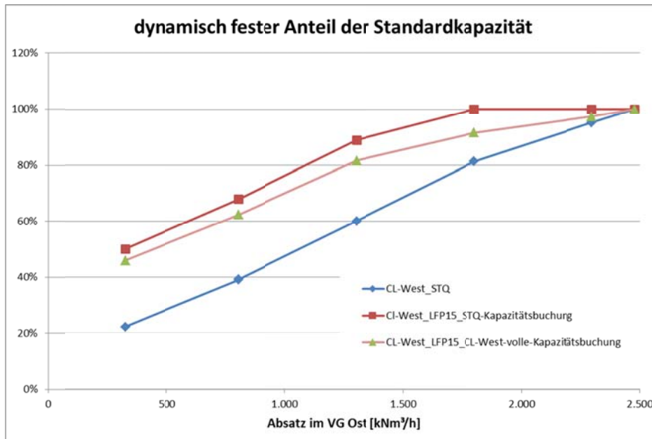
Diagramm 18: Dynamisch fester Anteil der Standardkapazität für den hydraulischen Cluster West im Status Quo und bei Umsetzung der genehmigten Projekte
