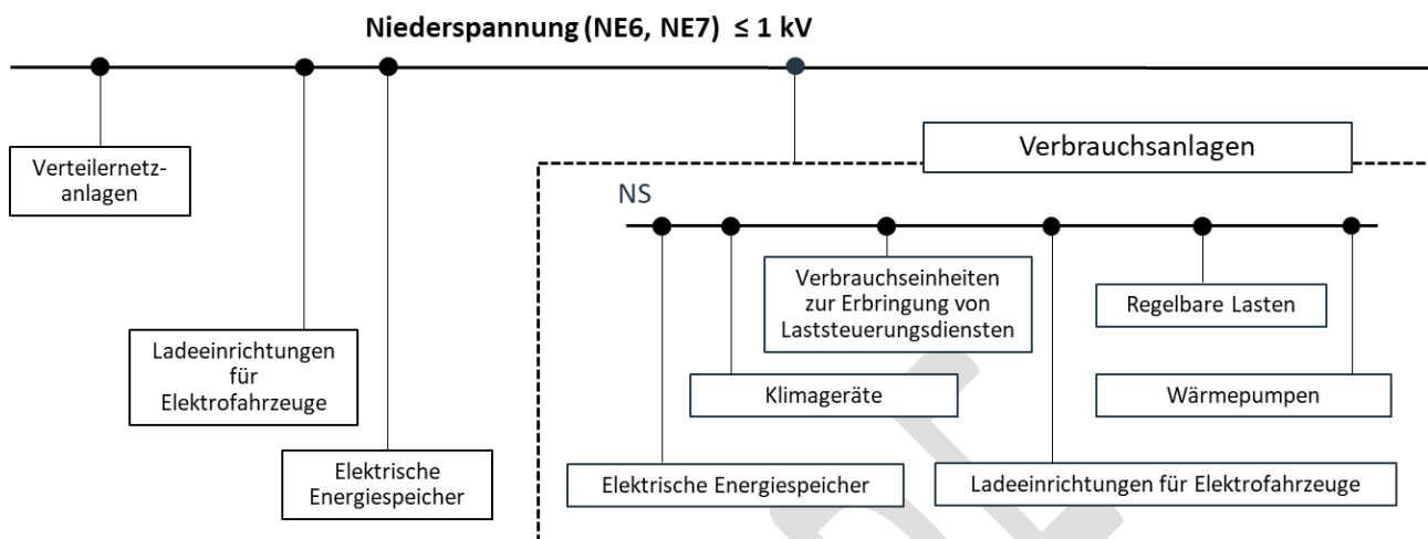
Abbildung 1: Übersicht Anwendungsbereich Mittelspannung (NE 6, NE 7)
