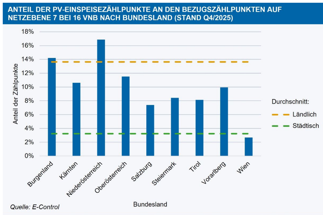
Abbildung 13: Anteil der Zählpunkte (Netzebene 7) für Photovoltaikanlagen an den Bezugszählpunkten bei 16 VNB in Q4/2025
