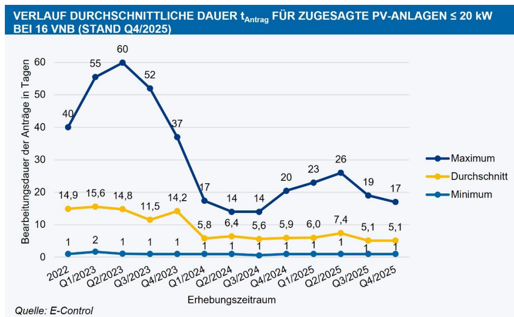
Abbildung 11: Verlauf der durchschnittlichen Zeitdauer t_{\text{Antrag}} für PV-Anlagen ≤ 20 kW Anlagenleistung bei 16 VNB, Stand Q4/2025 (zugesagte Anträge)
