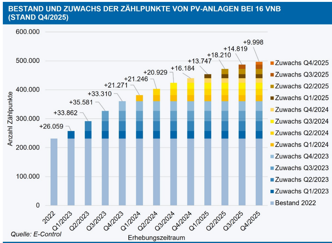
Abbildung 3: Entwicklung der Anzahl der Zählpunkte für Photovoltaik ab 2022 bei 16 VNB, Stand Q4/2025
