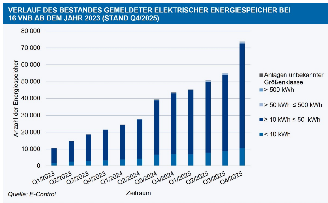
Abbildung 14: Verlauf des Bestandes gemeldeter elektrischer Energiespeicher bei 16 VNB ab dem Jahr 2023, Stand Q4/2025
