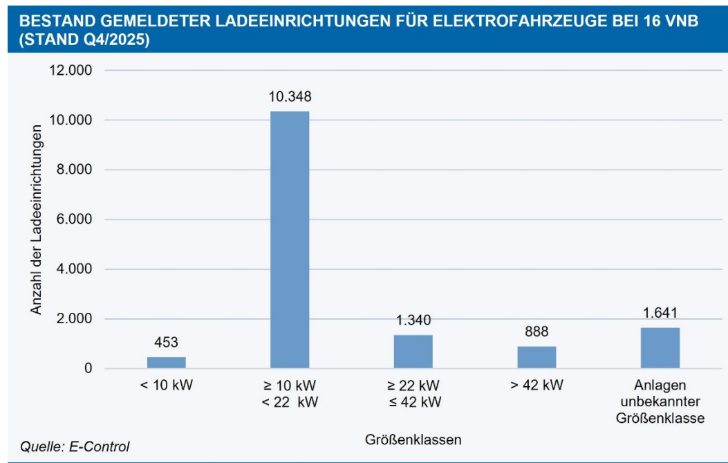
Abbildung 16: Bestand gemeldeter Ladeeinrichtungen für Elektrofahrzeuge bei 16 VNB, Stand Q4/2025
