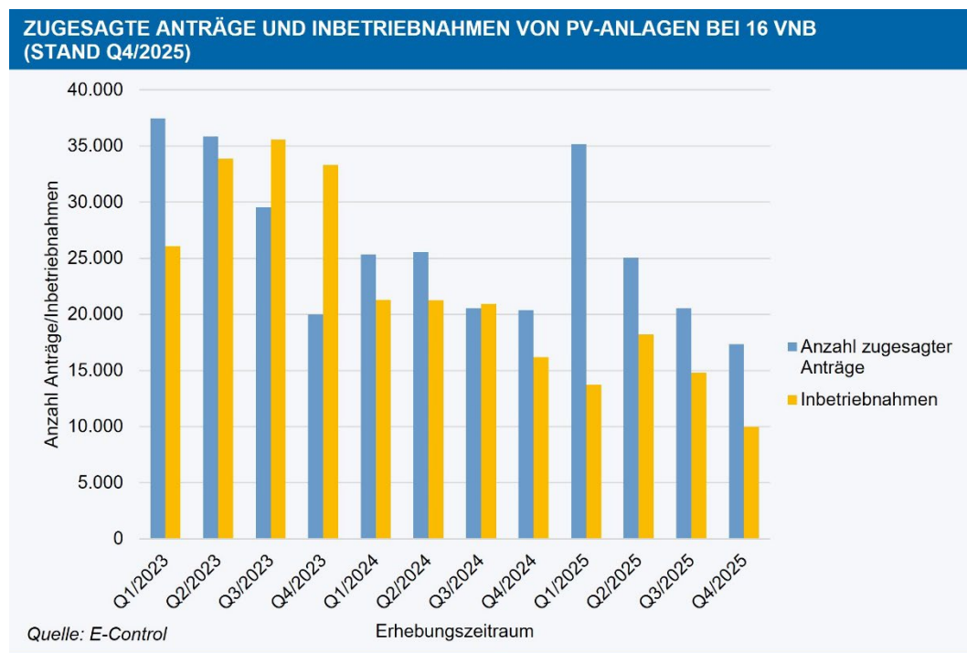
Abbildung 7: Zugesagte Anträge und neue Inbetriebnahmen von Photovoltaikanlagen bei 16 VNB ab 2023, Stand Q4/2025
