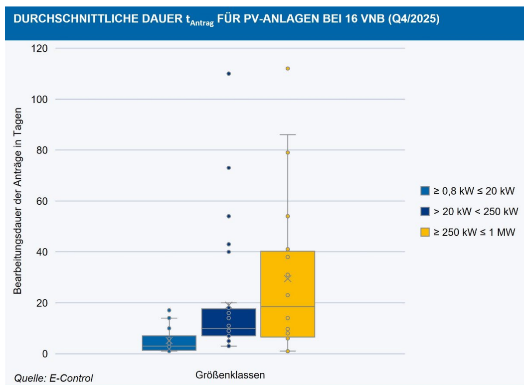
Abbildung 10: Durchschnittliche Bearbeitungsdauer der Anträge ( t_{\text{Antrag}} ) für PV-Anlagen über alle vollständigen Anträge, die bei den 16 VNB in Q4/2025 eingelangt sind.
