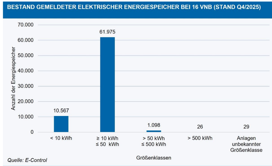
Abbildung 15: Bestand gemeldeter elektrischer Energiespeicher bei 16 VNB, Stand Q4/2025
