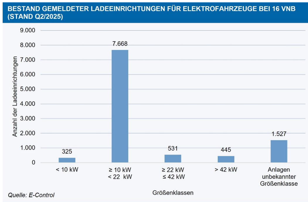
Abbildung 16: Bestand gemeldeter Ladeeinrichtungen für Elektrofahrzeuge bei 16 VNB, Stand Q2/2025
