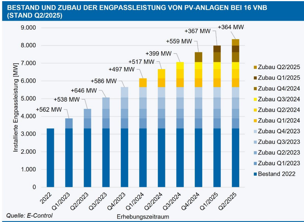
Abbildung 2: Entwicklung des Bestands und des Zubaus von Photovoltaik ab 2022 bei 16 VNB, Stand Q2/2025
