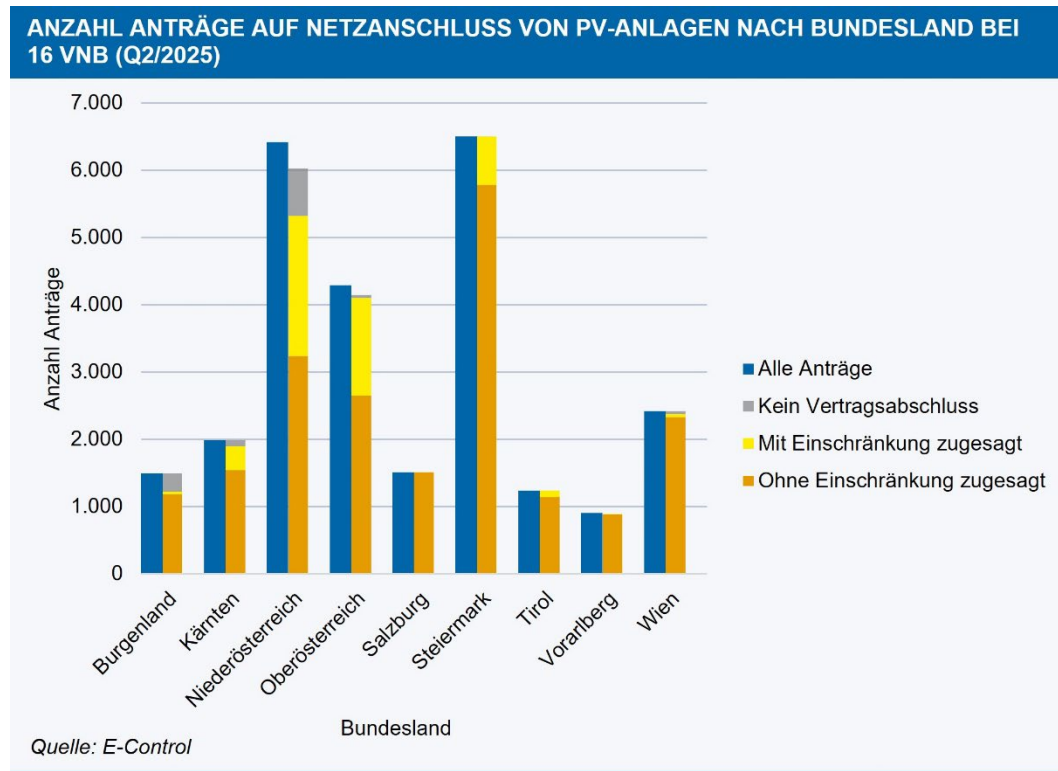
Abbildung 6: Anträge auf Netzanschluss für PV-Anlagen bei 16 VNB pro Bundesland in Q2/2025
