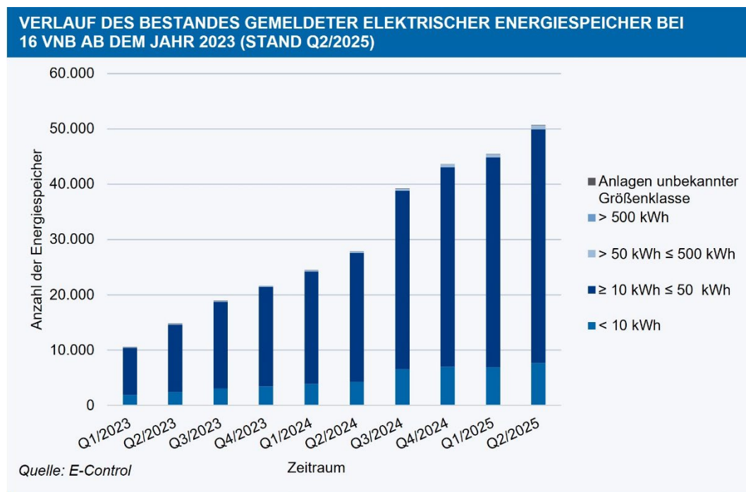
Abbildung 14: Verlauf des Bestandes gemeldeter elektrischer Energiespeicher bei 16 VNB ab dem Jahr 2023, Stand Q2/2025
