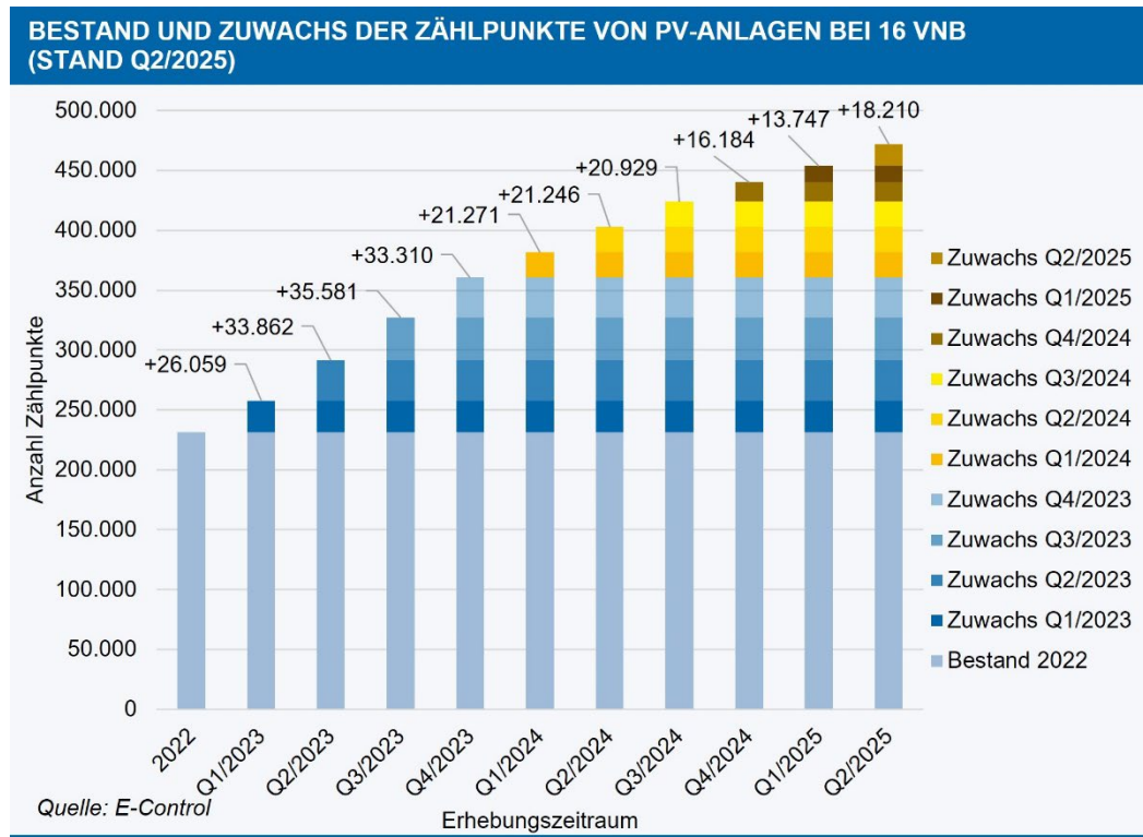
Abbildung 3: Entwicklung der Anzahl der Zählpunkte für Photovoltaik ab 2022 bei 16 VNB, Stand Q2/2025
