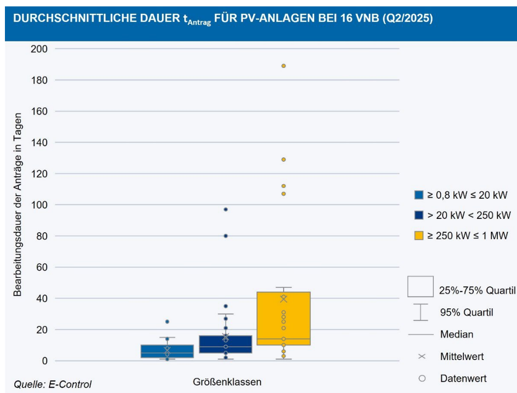
Abbildung 10: Durchschnittliche Bearbeitungsdauer der Anträge ( t_{\text{Antrag}} ) für PV-Anlagen über alle vollständigen Anträge, die bei den 16 VNB in Q2/2025 eingelangt sind.
