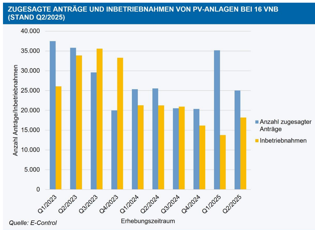
Abbildung 7: Zugesagte Anträge und neue Inbetriebnahmen von Photovoltaikanlagen bei 16 VNB ab 2023, Stand Q2/2025
