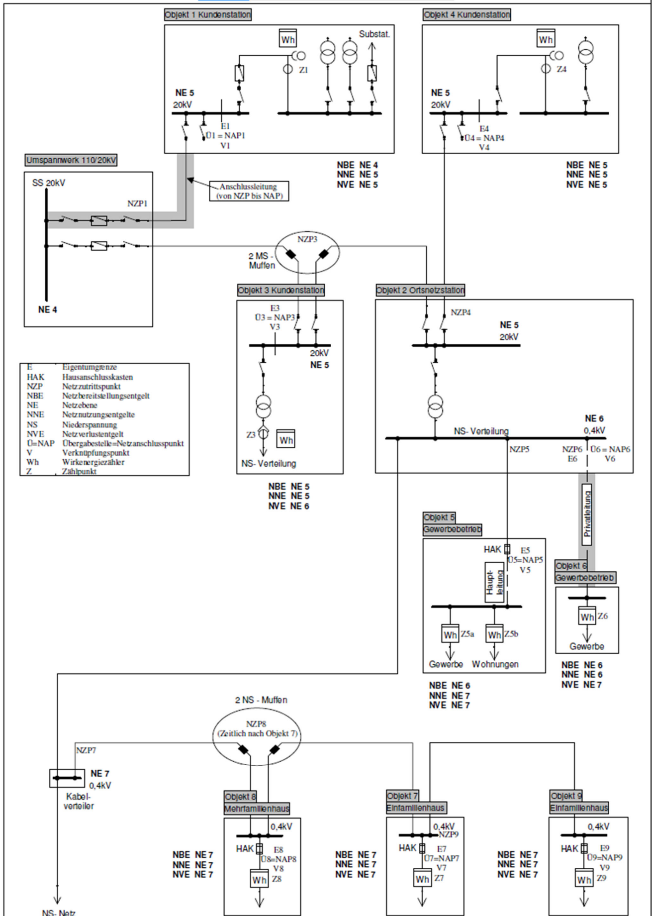
Abbildung 10: Schema Bezugspunkte in Verteilernetzen
