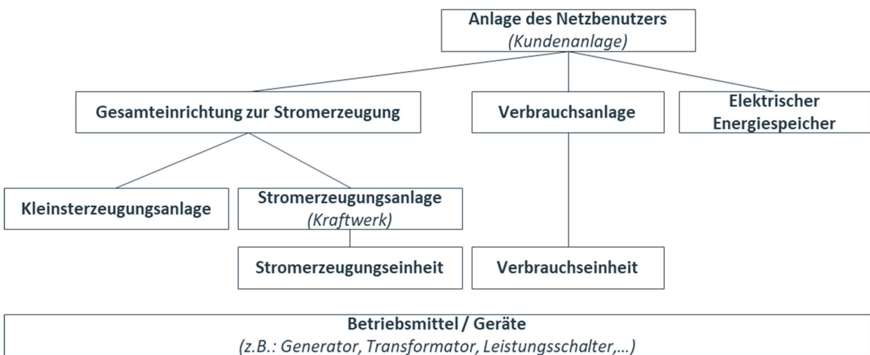
Abbildung 2: Schema Anlagenbegriffe Netzbennutzer
