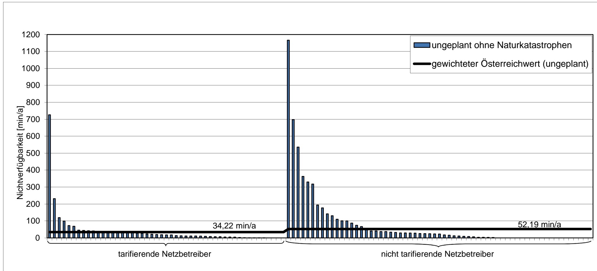
Abbildung 7: Ungeplante Nichtverfügbarkeit (ASIDI) für die Netze der erhobenen tarifizierenden und nicht tarifizierenden Netzbetreiber im Jahr 2012 und den jeweiligen bezogenen gewichteten Nichtverfügbarkeitswerten (34,22 min bzw. 52,19 min)
