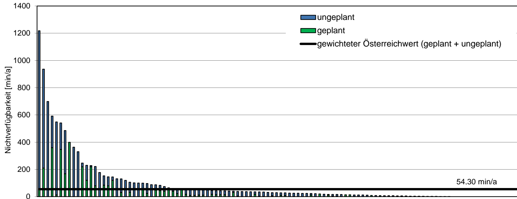
Abbildung 6: Nichtverfügbarkeit (ASIDI) der österreichischen Mittelspannungsnetze im Jahr 2012, unterschieden nach geplanten und ungeplanten Versorgungsunterbrechungen und gewichtetem Österreichwert (54,30 min)
