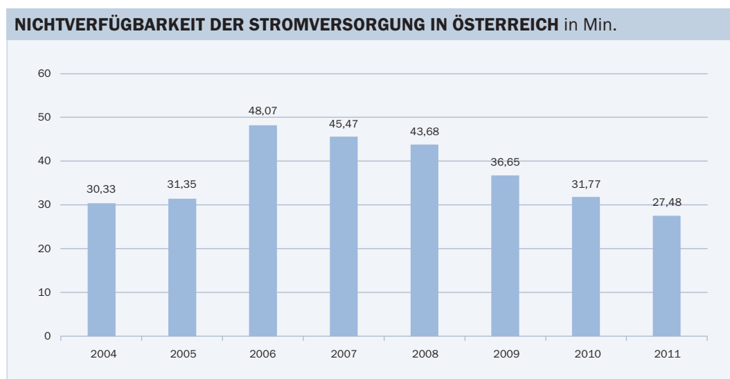
Abbildung 25 Jährliche ungeplante Nichtverfügbarkeit (ASIDI) der Stromversorgung in Österreich
