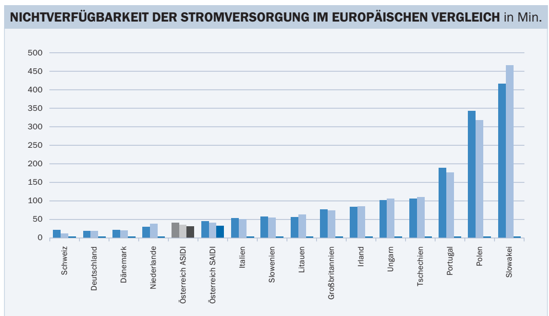
Abbildung 26 Jährliche Nichtverfügbarkeit der Stromversorgung in Mittelspannungsnetzen im europäischen Vergleich (SAIDI, nur für Österreich auch ASIDI) 18
