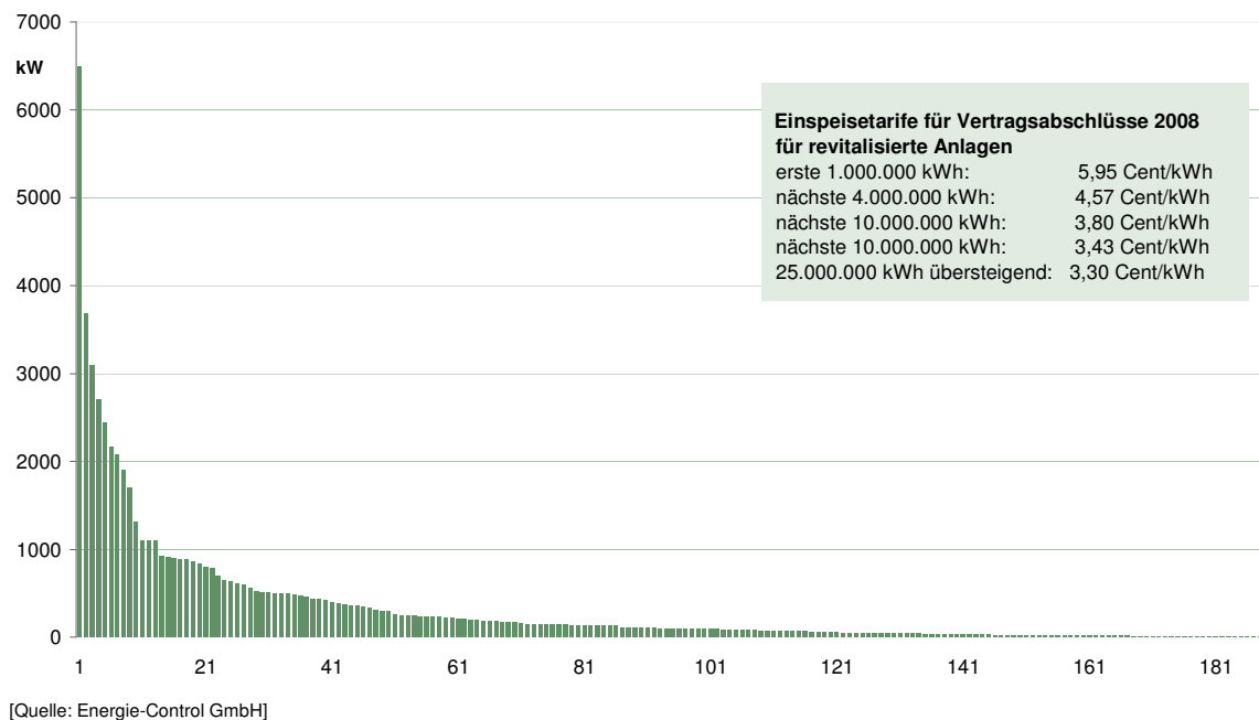
Abbildung 25: Anerkannte revitalisierte Kleinwasserkraft-Anlagen, Revitalisierung > 15 %, (Summe: 189 Anlagen, 63 MW) im Größenvergleich per Ende des 4. Quartals 2008
