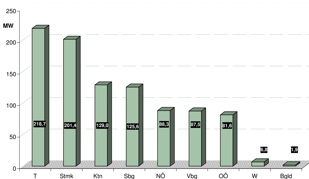
Abbildung 17: Anerkannte bestehende Kleinwasserkraft-Anlagen (Altanlagen) nach Bundesländern, Stand 31.12.2008
