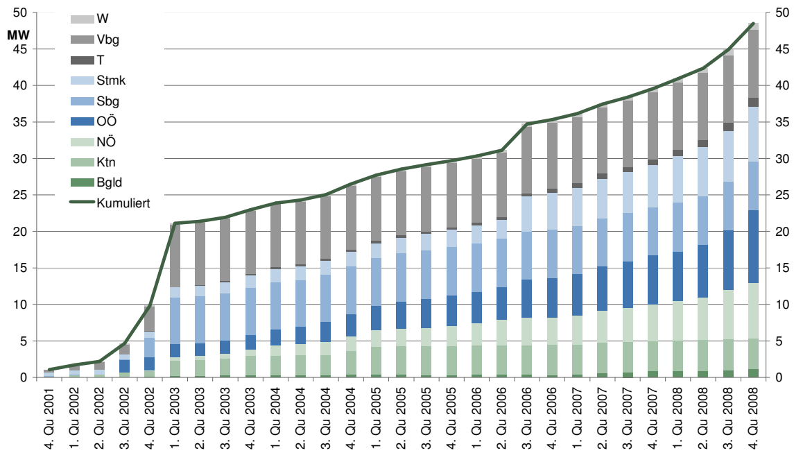
Abbildung 52: Entwicklung anerkannter Photovoltaik-Anlagen vom 4. Quartal 2001 - 4. Quartal 2008
