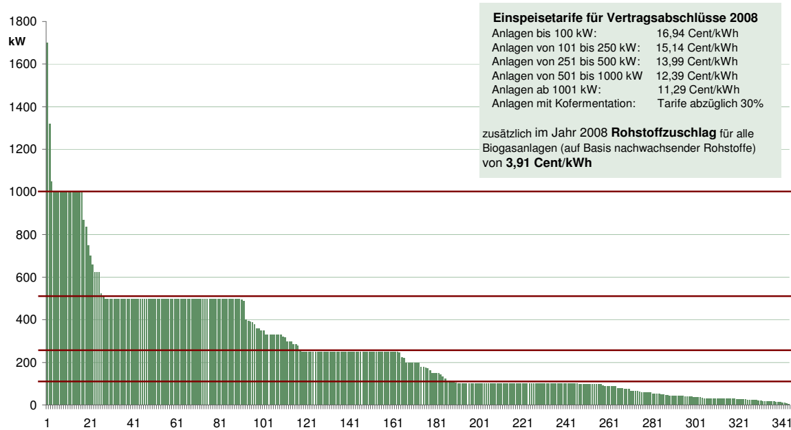
Abbildung 36: Anerkannte Biogasanlagen (Summe: 344 Anlagen, 92,1 MW) im Größenvergleich per Ende des 4. Quartal 2008
