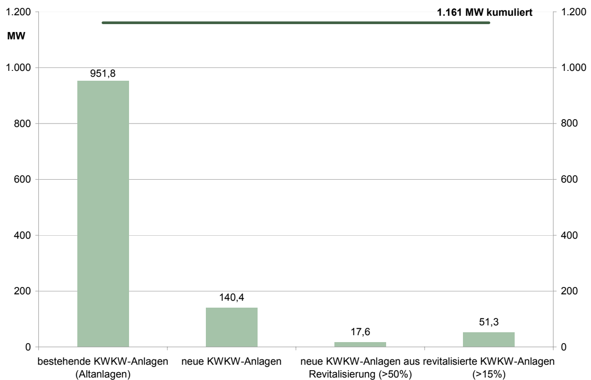
Abbildung 42: Kleinwasserkraft-Leistungssummen für unverändert bestehende, revitalisierte (unvollständig) und neue Kleinwasserkraft-Anlagen per Ende des 1. Quartals 2007
