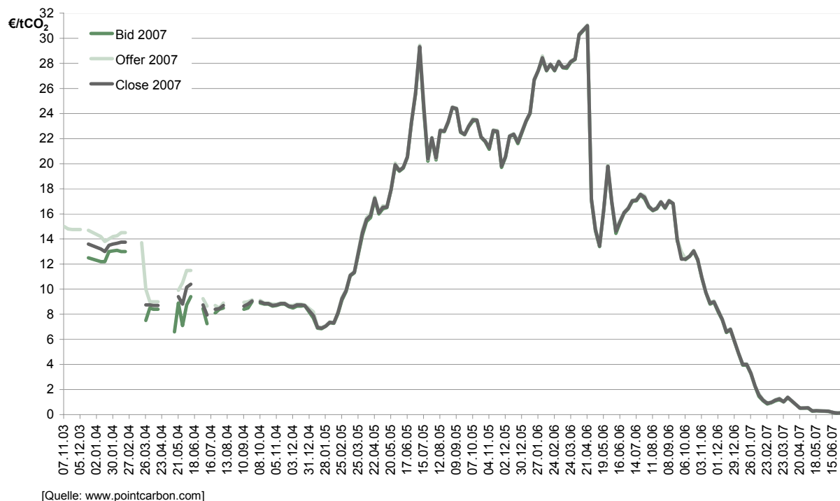
Abbildung 35: CO 2 (EU-ETS 2007) - Preisentwicklung 07.11.2003 - 30.06.2007
