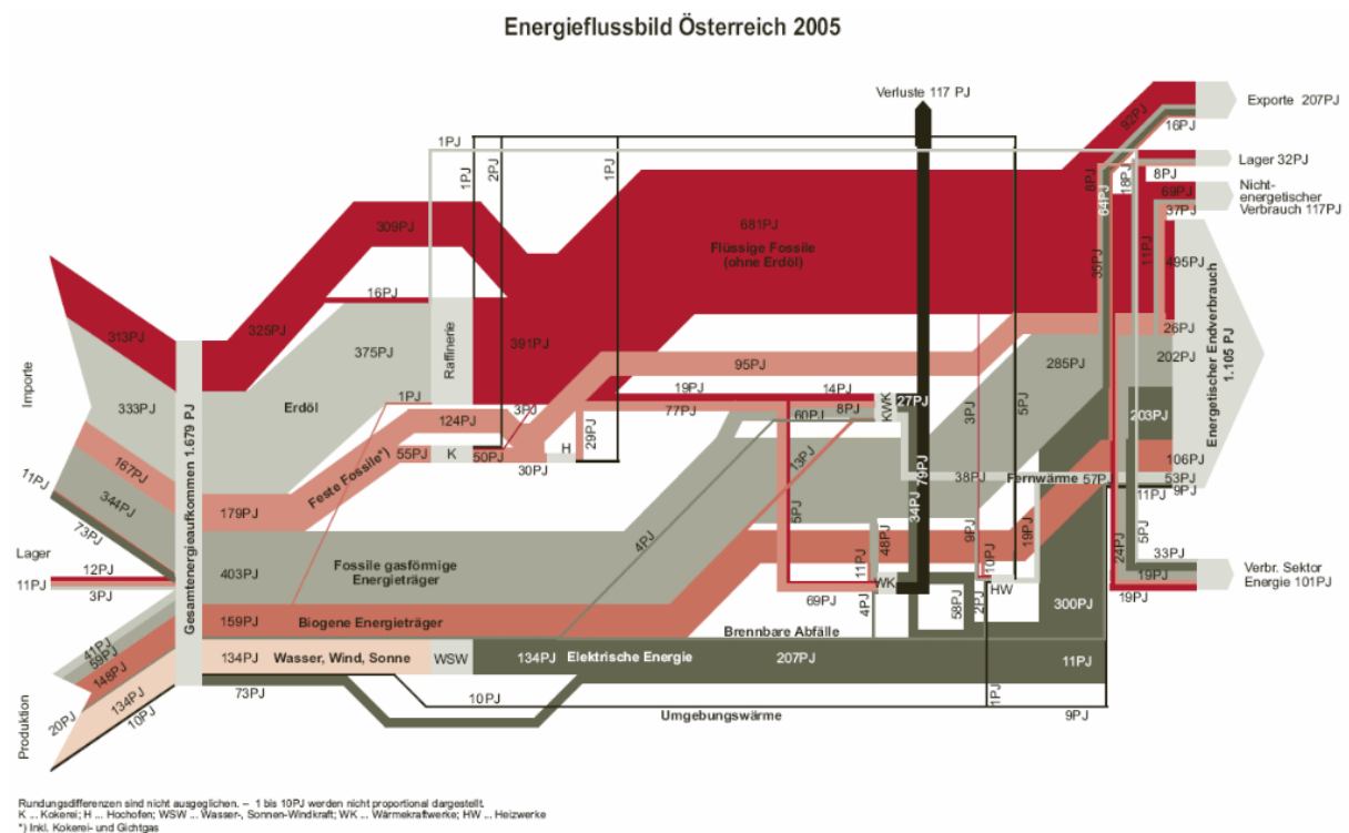
Abbildung 8: Energieflussbild 2005
