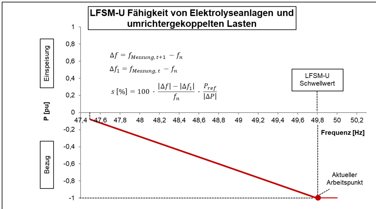
Abbildung 5: Fähigkeit von Elektrolyseanlagen und unrichtergekoppelten Lasten zur frequenzabhängigen Anpassung der Wirkleistung im LFSM-U-Modus (Darstellung für P_{\text{ref}} = P_{\text{mom}} und s = 5\% )
